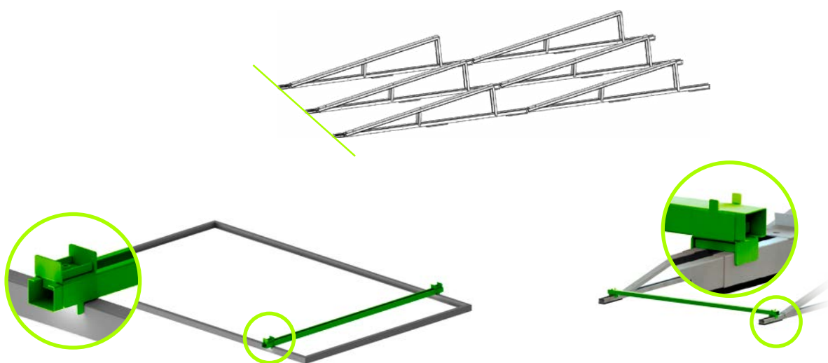
Setați lățimea panoului pe distanțier.
